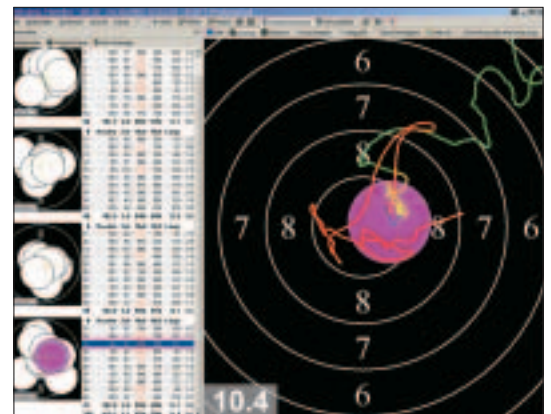
SCATT-Zielwegdarstellung
